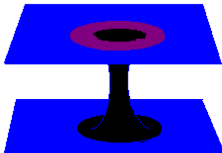
Cunicolo spazio-tempo, che collega due universi paralleli
